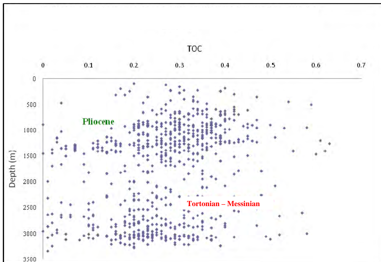
Figure 2. Content of organic carbon (TOC) vs depth in Miocene-Pliocene deposits from Dvjaka anticline. Figura 2. Conținutul de carbon organic (TOC) versus adâncime în depozitele miocen-pleiocene din zona Divjaka.
