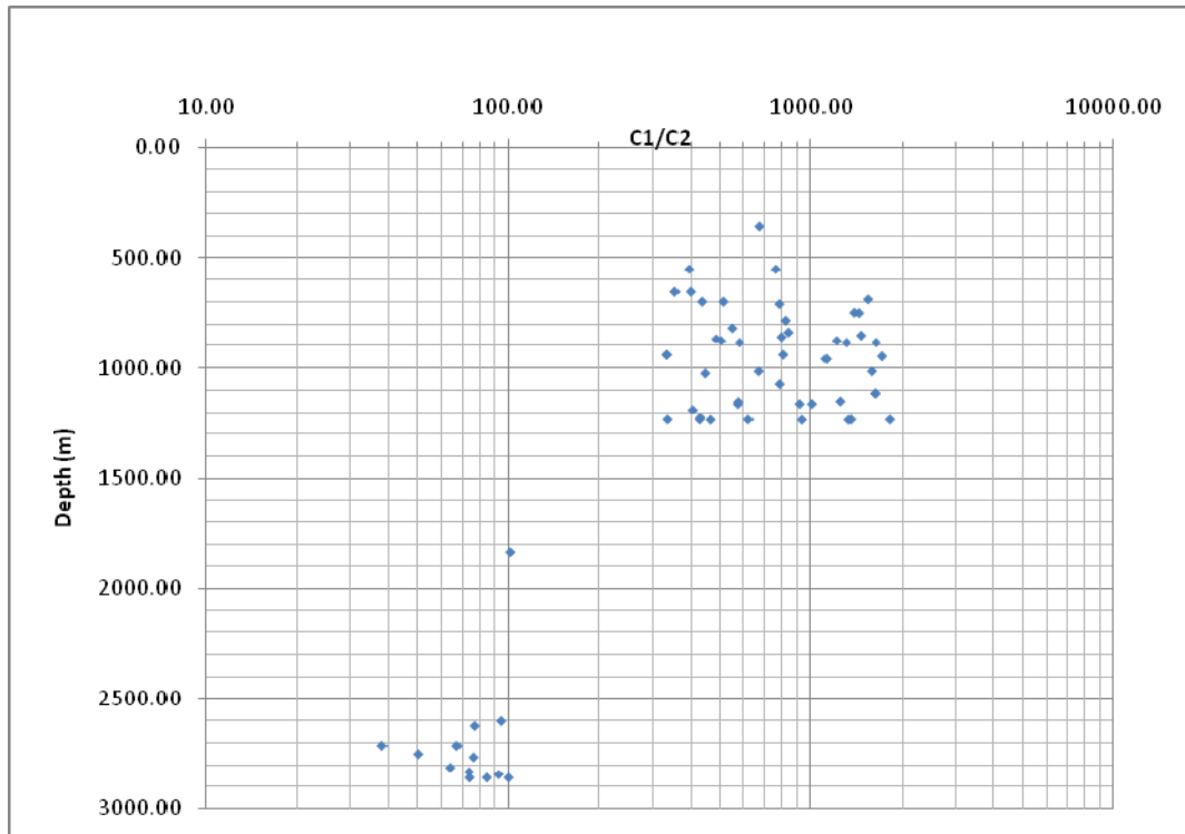
Figure 5. C_1/C_2 vs depth, in deeper section generated wet gas. Figura 5. C_1/C_2 versus adâncime în secțiune mai adâncă generează gaz umed.
