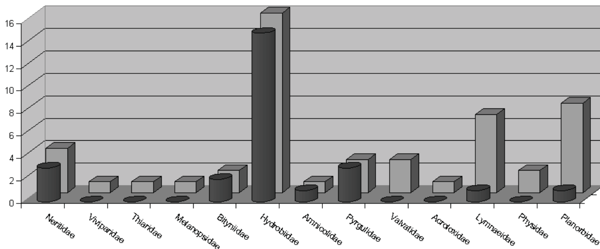
Figure 1. Comparison of endemic (front row) and total nominal taxa for each families. Figura 1. Comparație între taxonii endemici și numărul total de taxoni ai fiecărei familii.
